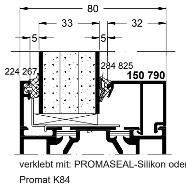
Al.-Blech t = 2; 3 × Gipskartonplatte (GKB) t=9,5
